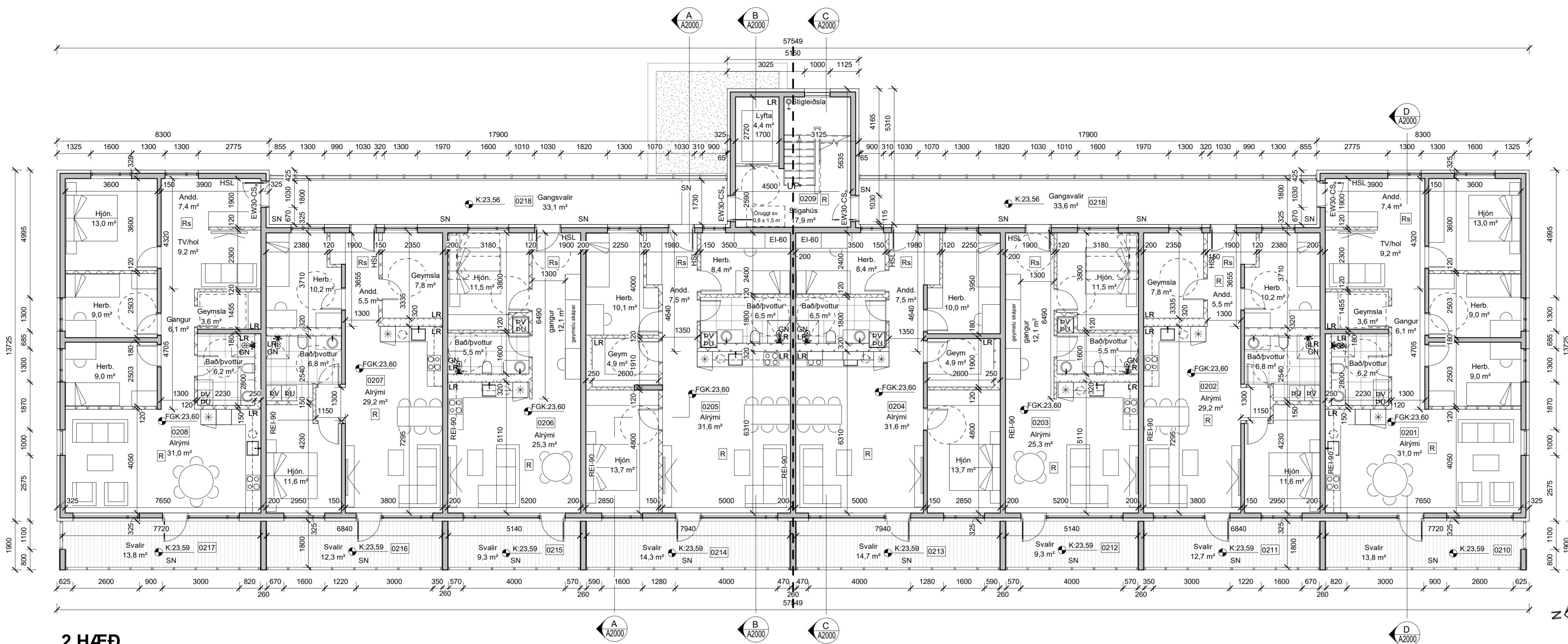
2. HÆÐ mkv: 1 : 100
