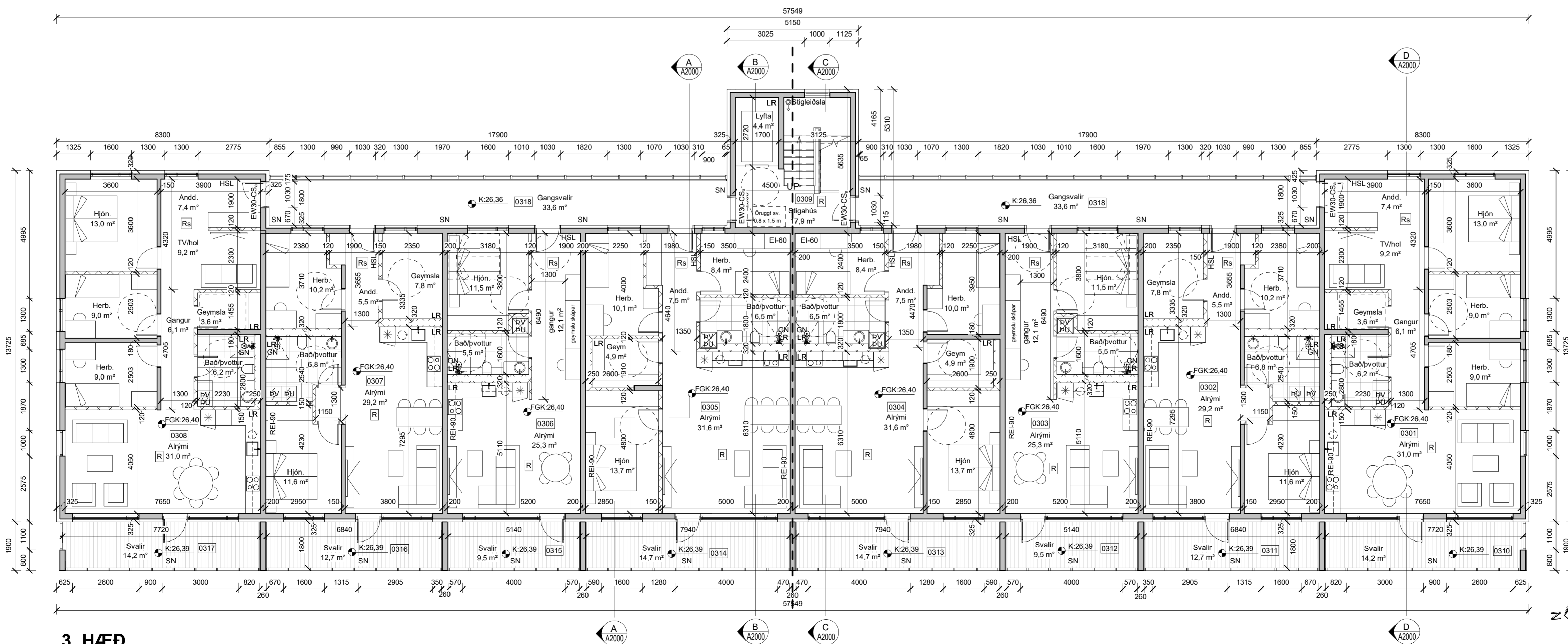
3. HÆÐ mkv: 1 : 100
