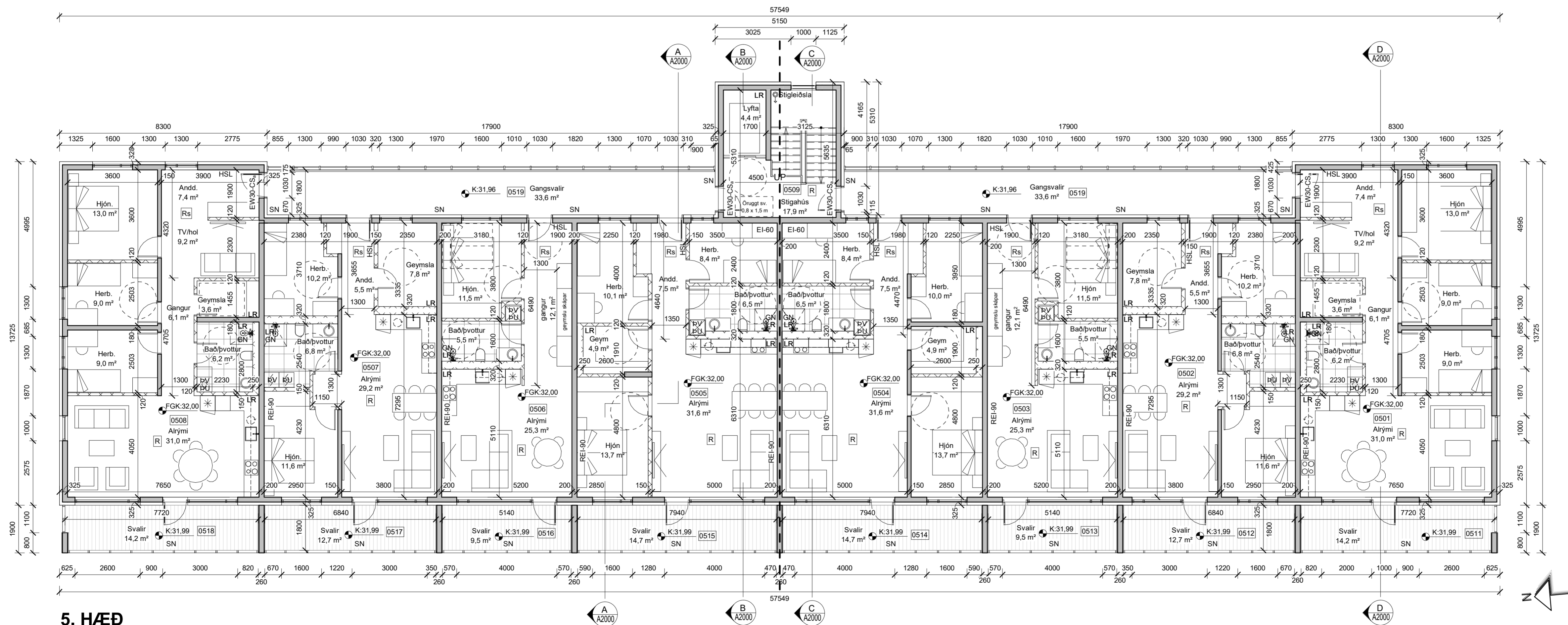
5. HÆÐ mkv: 1 : 100
