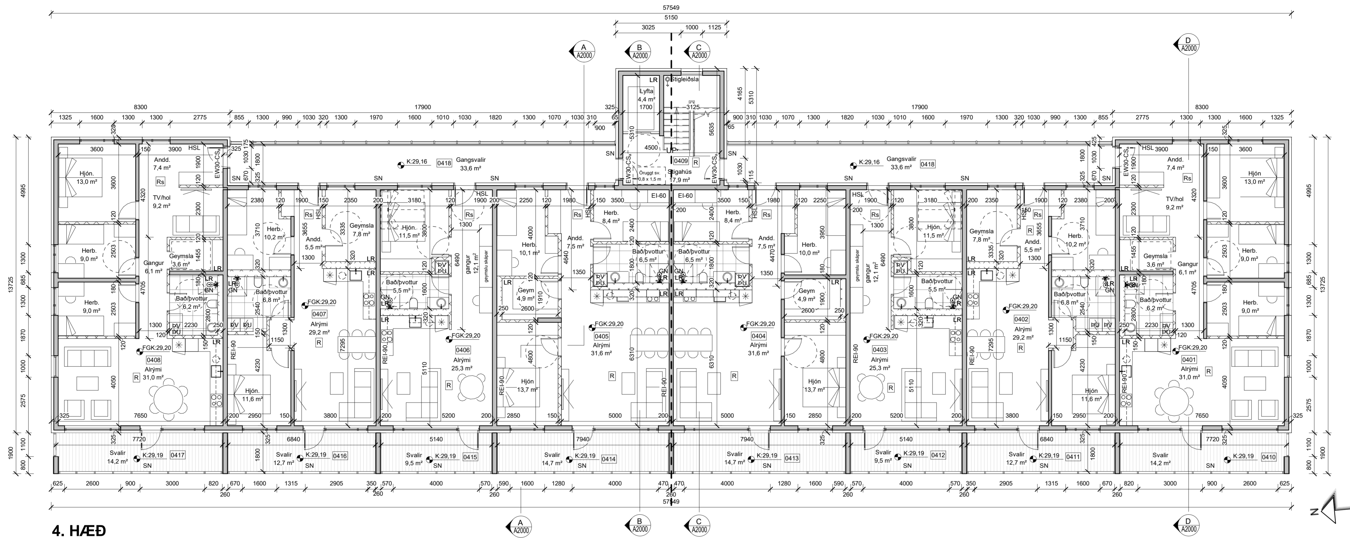
4. HÆÐ mkv: 1 : 100
